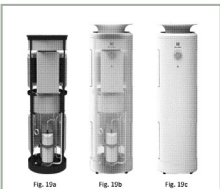
Struttura del prodotto: forma circolare/conica.
