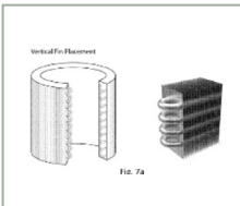
Scambiatore di calore cilindrico.
